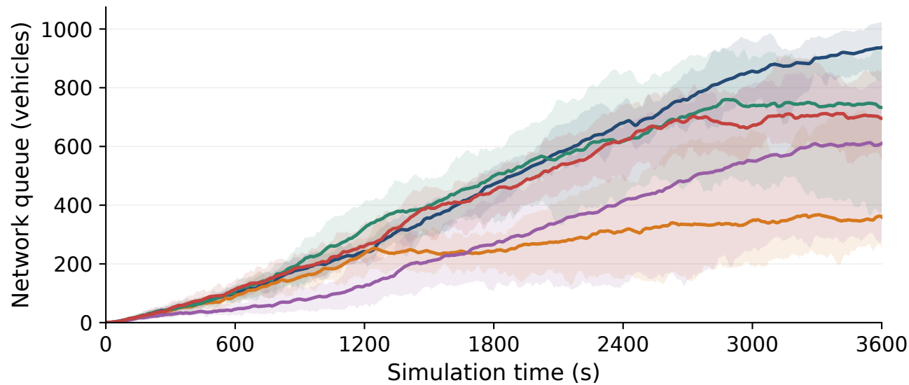
IQLL
